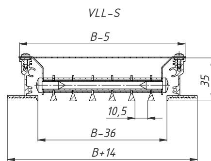
Сечение решетки
