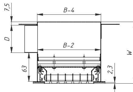
Сечение решетки
